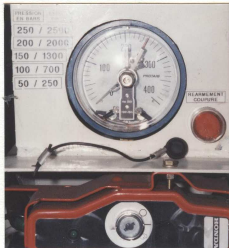
DYNAMOMETEUR HEP.i DC2.5
